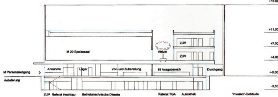
Längsschnitt A-A
