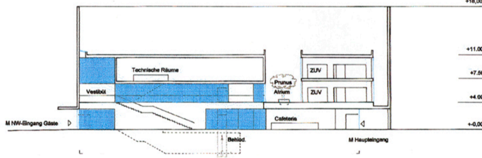
Querschnitt C-C
