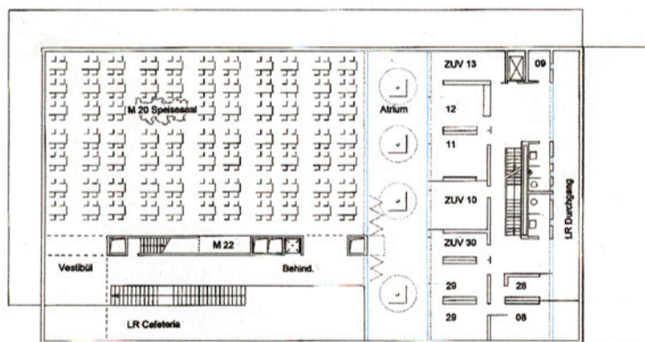
1. Obergeschoss
