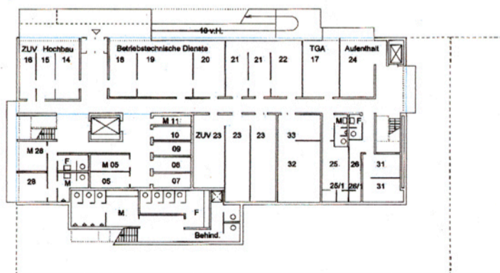
Untergeschoss
