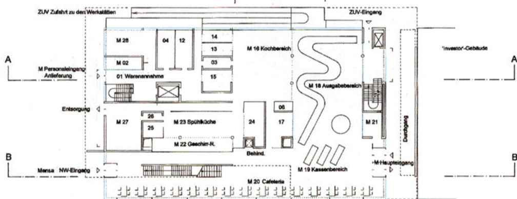
Erdgeschoss
