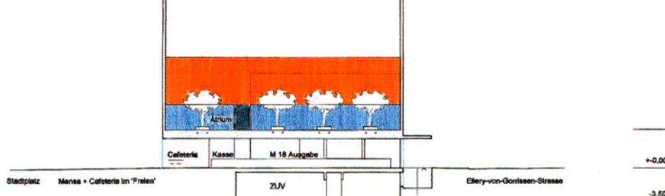
Querschnitt D-D
